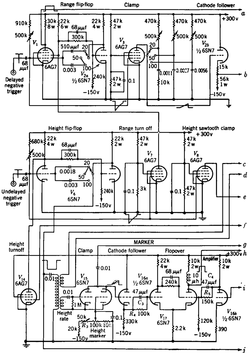
FIG. 15-7.—Range-height
